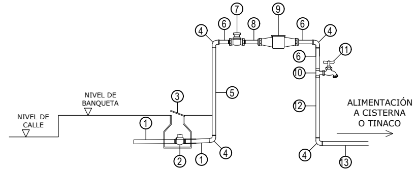
No. CONCEPTO CANT. UNIDAD 1 NIPLE DE Fo.Go. C-40 DE ½" DE Ø CON LONG. DE 20 CMS 2 PZA 2 LLAVE DE BANQUETA DE 13 MM Ø 1 PZA 3 BOTA DE FO.FO. P/LLAVE DE BANQUETA 1 PZA 4 CODO DE Fo.Go. DE 90° x ½" DE Ø 4 PZA 5 NIPLE DE Fo.Go. C-40 DE ½" DE Ø CON LONG. DE 80 CMS 1 PZA 6 NIPLE DE Fo.Go. C-40 DE ½" DE Ø CON LONG. DE 5 MCS 6 PZA 7 VALVULA DE ESFERA ANTIGRAUDE DE ½" DE Ø 1 PZA 8 NIPLE DE Fo.Go. C-40 DE ½" DE Ø CON LONG. DE 10 MCS 1 PZA 9 MEDIDOR DE AGUA POTABLE DE ½" DE Ø 1 PZA 10 TEE DE Fo.Go. C-40 DE ½" DE Ø (OPCIONAL) 1 PZA 11 LLAVE DE JARDIN DE ½" DE Ø DE BRONCE (OPCIONAL) 1 PZA 12 NIPLE DE Fo.Go. C-40 DE ½" DE Ø CON LONG. DE 70 MCS 1 PZA 13 TUBERIA DE Fo.Go. C-40 DE ½" DE Ø CON LONG. DE VARIABLE 1 PZA
